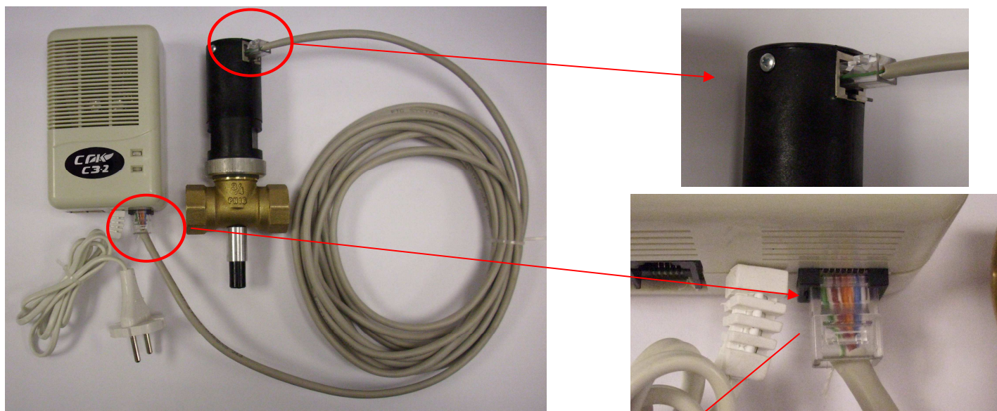
Рисунок 12. Система автономного контроля загазованности СГК-1-СО(слева). Справа показаны разъемы RJ-45на клапане (рис. вверху справа) и на сигнализаторе (внизу справа).
