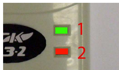
Рисунок 21. Индикаторы сигнализатора СЗ-2. Авария «обрыв клапана».
