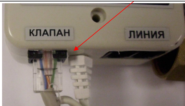
Рисунок 13. Вид на разъем RJ-45на сигнализаторе со стороны задней панели. (кабель подключен)
