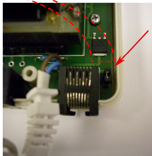
Рисунок 11. Сигнализатор СЗ-2. Имитатор клапана включен.
