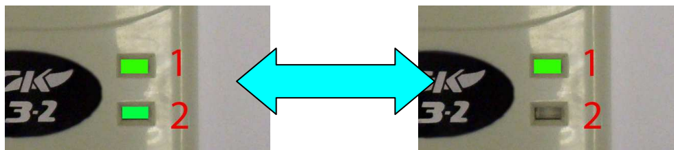
Рисунок 20. Индикаторы сигнализатора СЗ-2. Авария «обрыв связи».
