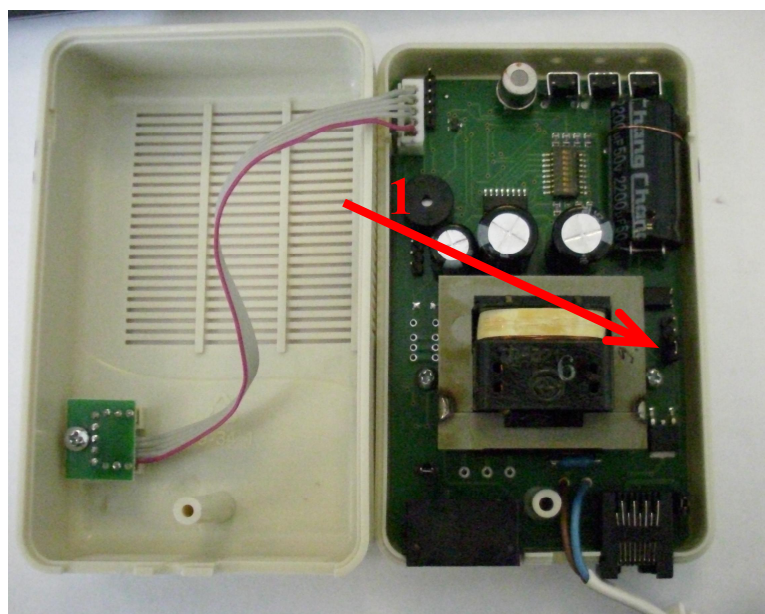
Рисунок 8. Сигнализатор СЗ-Х. 1- перемычка, включающая режим энергонезависимой системы.
