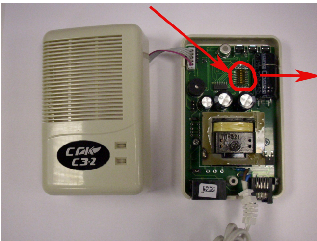
Рисунок 5. Сигнализатор СЗ-Х. Вид со снятой передней панелью. Стрелками отмечено расположение микропереключателей адреса
