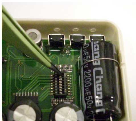
Рисунок 7. Переключение адреса.
