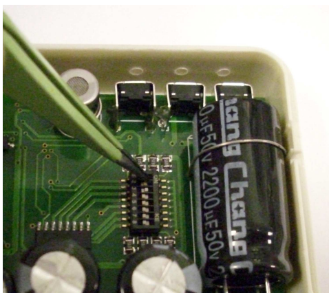
Рисунок 7. Переключение адреса.
