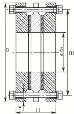
Рисунок 3 - Изолирующее фланцевое соединение ИФС-Б
